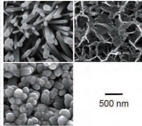
水溶液プロセスにより作製した生体活性の高い水酸アパタイト系皮膜の表面写真 Surface photo of a hydroxyapatite coating with a high bioactivity prepared by solution processing
