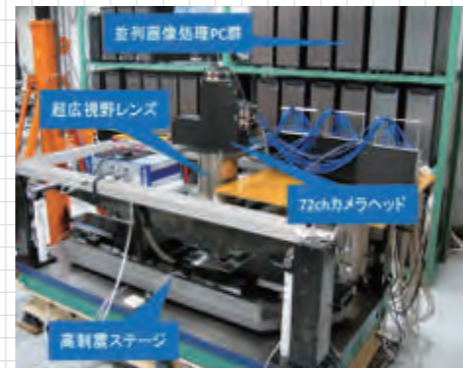
超高速原子核乾板読み出し装置 Hyper Track Selector
