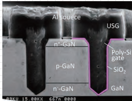
GaNトレンチMOSFETの断面写真(豊田中研/トヨタ共同開発) Cross-sectional TEM of GaN trench MOSFET
