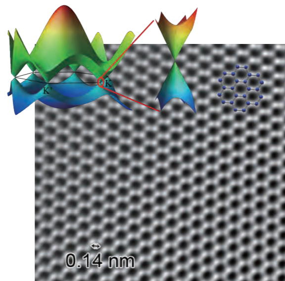
エピタキシャルグラフェンの高分解能TEM像および逆空間におけるバンド構造の線形分散関係 High resolution transmission electron microscopy image of epitaxial graphene and the linear dispersion relation of graphene band structure
