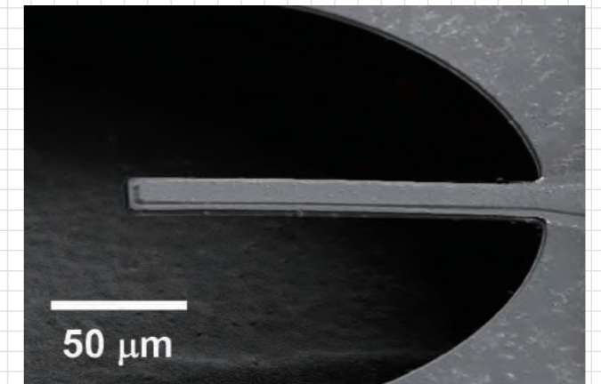
カンチレバー形状に微細加工した(K,Na)NbO 3 系無鉛圧電セラミックス薄膜の電子顕微鏡写真 Scanning electron micrograph of lead-free piezoelectric (K,Na)NbO 3 -based thin film microfabricated in cantilever shape
