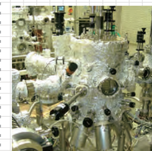
8元マグネトロンスputタ装置 Magnetron sputtering with 8 sources
