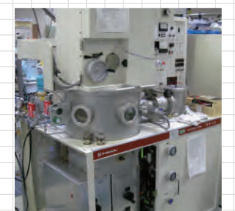
3元マグネトロンスputタ装置 Magnetron sputtering with 3 sources
