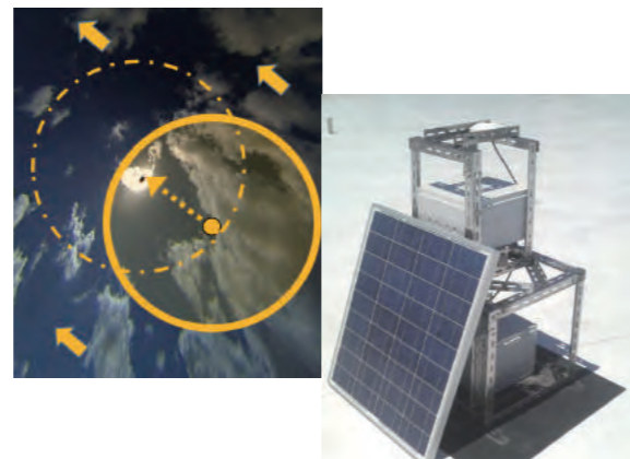
全天画像を用いた配電エリアにおける太陽光発電の把握・予測システム Nowcasting/Forecasting System of Photovoltaic Power Generation in Distribution Network using All-sky Images
