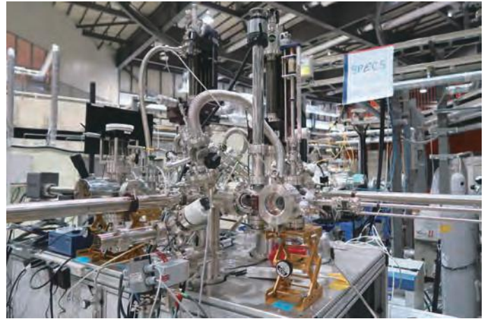
あいちシンクロtron (BL6N1) の放射光 XAFS-XPS 分析装置 XAFS-XPS analysis system in Aichi SR (BL6N1)
