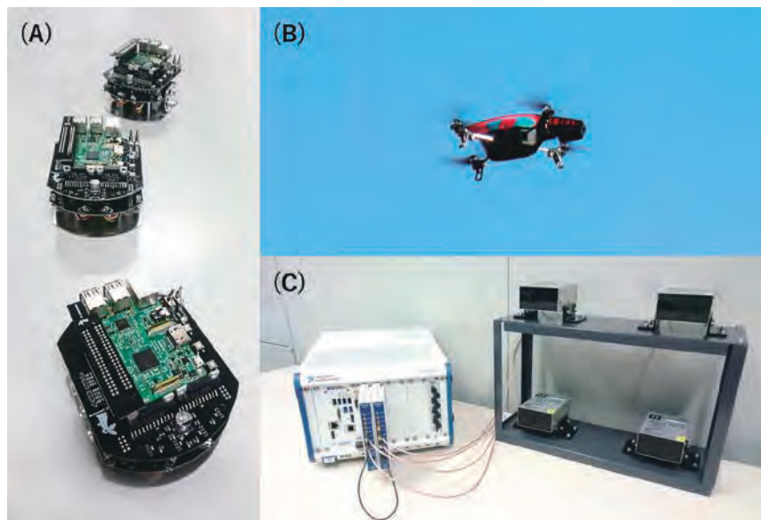
(A) 無線制御隊列走行 Wireless controlled platooning (B) ドローン無線ネットワーク Wireless drone network (C) 光無線 MIMO 通信 Optical wireless MIMO modem
