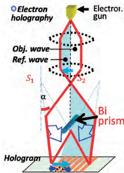
高分解能電子顕微鏡・ホログラフィーを用いた、動作状態のナノスケールトランジスタ内部のポテンシャル可視化 Direct electrostatic potential mapping in nano-scaled FET under operation mode using electron holography
