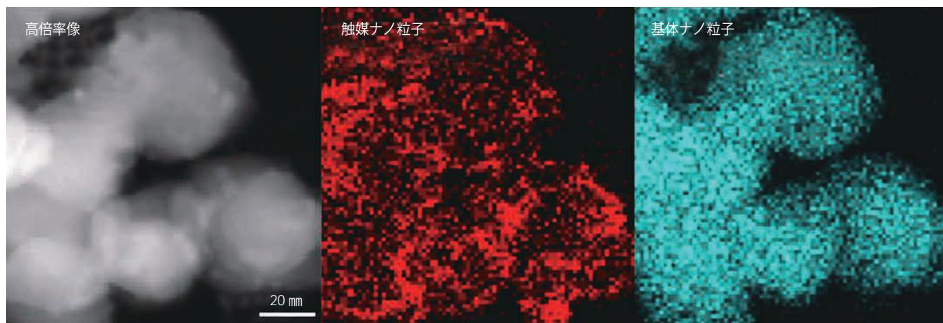
ナノ粒子の複合化による高性能な環境保全（排気浄化触媒）技術の開発（電子顕微鏡による元素分布の観察）
