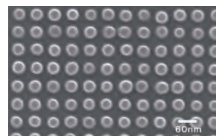
電子線描画によるナノパターン形成 Nano-pattern by EB lithography
