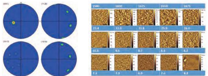
3つの核形成時間と様々なアニーリング温度で、有機金属気相成長法により形成されたAIN膜(10-10)面の原子間力顕微鏡画像。図中の数字は粗さ(nm)を示す。
