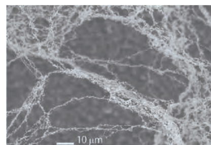
ヘリウムプラズマ照射により形成されたタングステンのナノワイヤー Tungsten nanowires grown by an exposure to a helium plasma.
