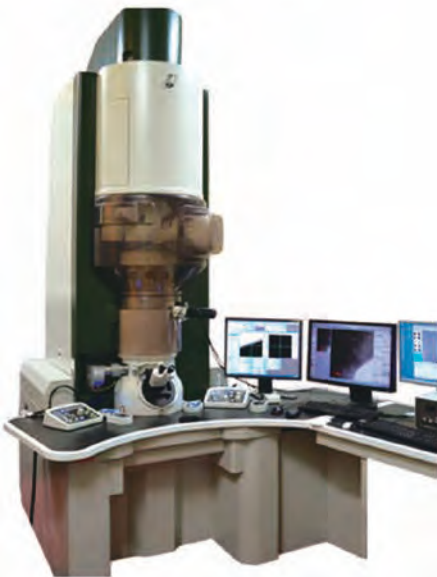
高分解能電子顕微鏡・ホログラフィーを用いた、動作状態のナノスケールトランジスタ内部のポテンシャル可視化 Direct electrostatic potential mapping in nano-scaled FET under operation mode using electron holography
